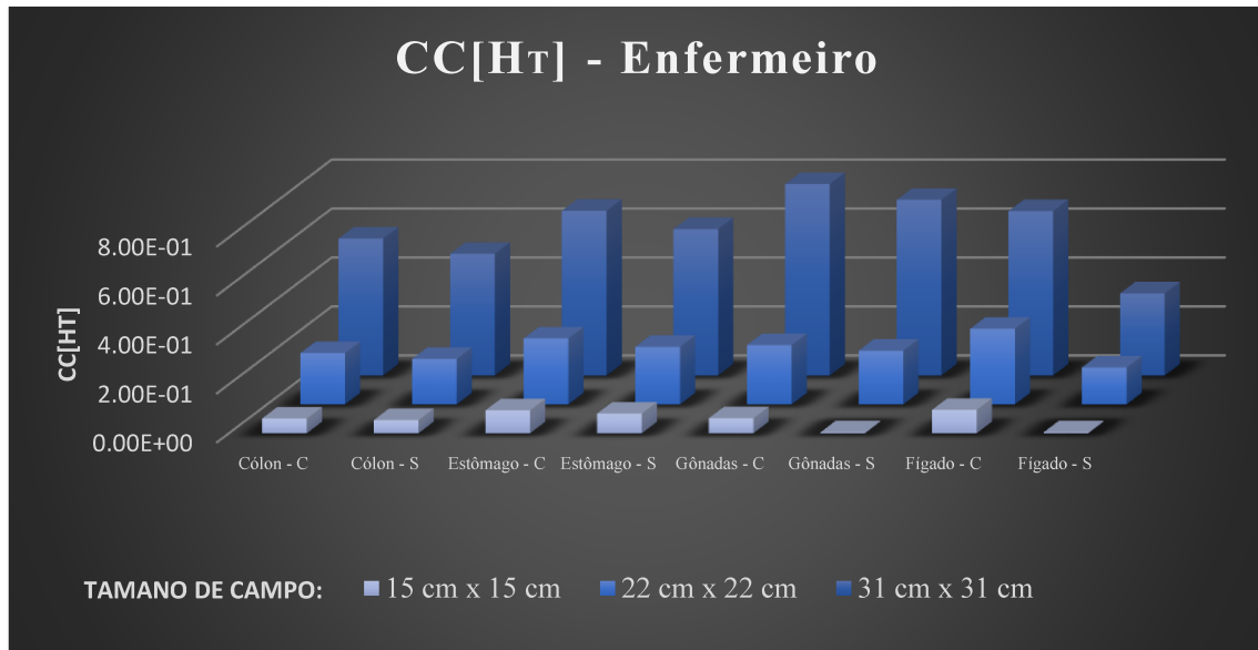
Figura 5 - Valores de CC[H_T]_{MASCULINO} em órgãos mais afetados no enfermeiro, considerando uma tensão no tubo de 100 kV. “C” significa avental com fissura e “S” sem fissura.
