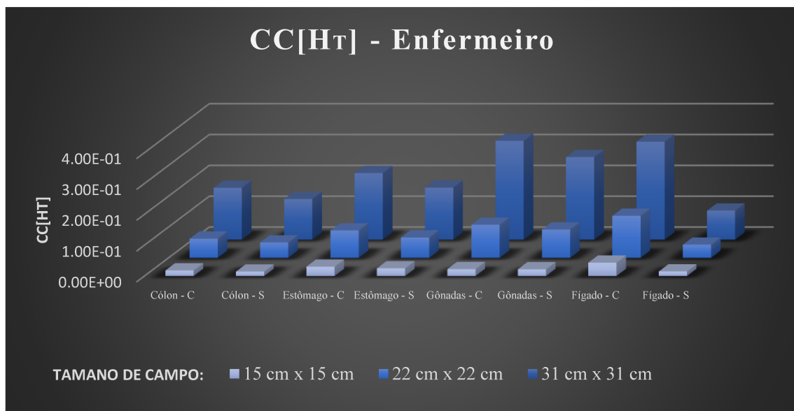
Figura 6 - Valores de CC[H_T]_{MASCULINO} em órgãos mais afetados no enfermeiro, considerando uma tensão no tubo de 80 kV. “C” significa avental com fissura e “S” sem fissura.
