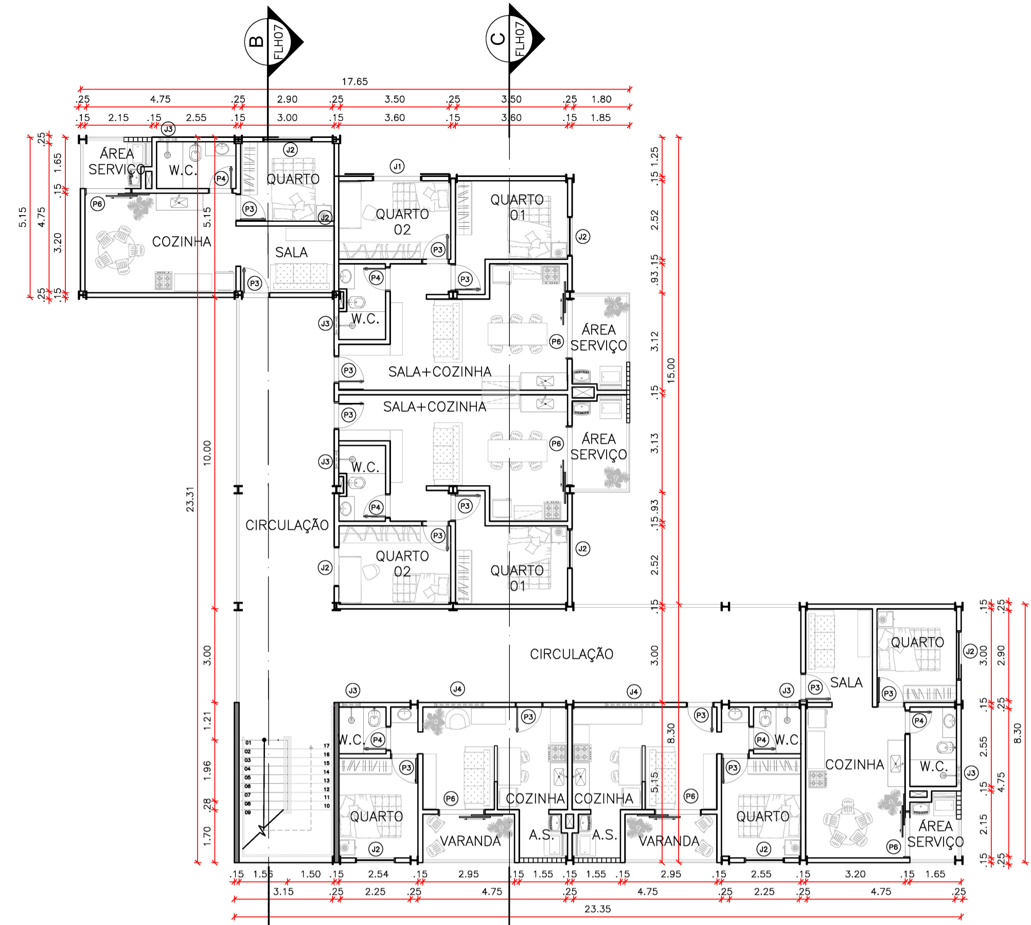
09 PAVIMENTO TIPO BLOCO C ESCALA 1:125
