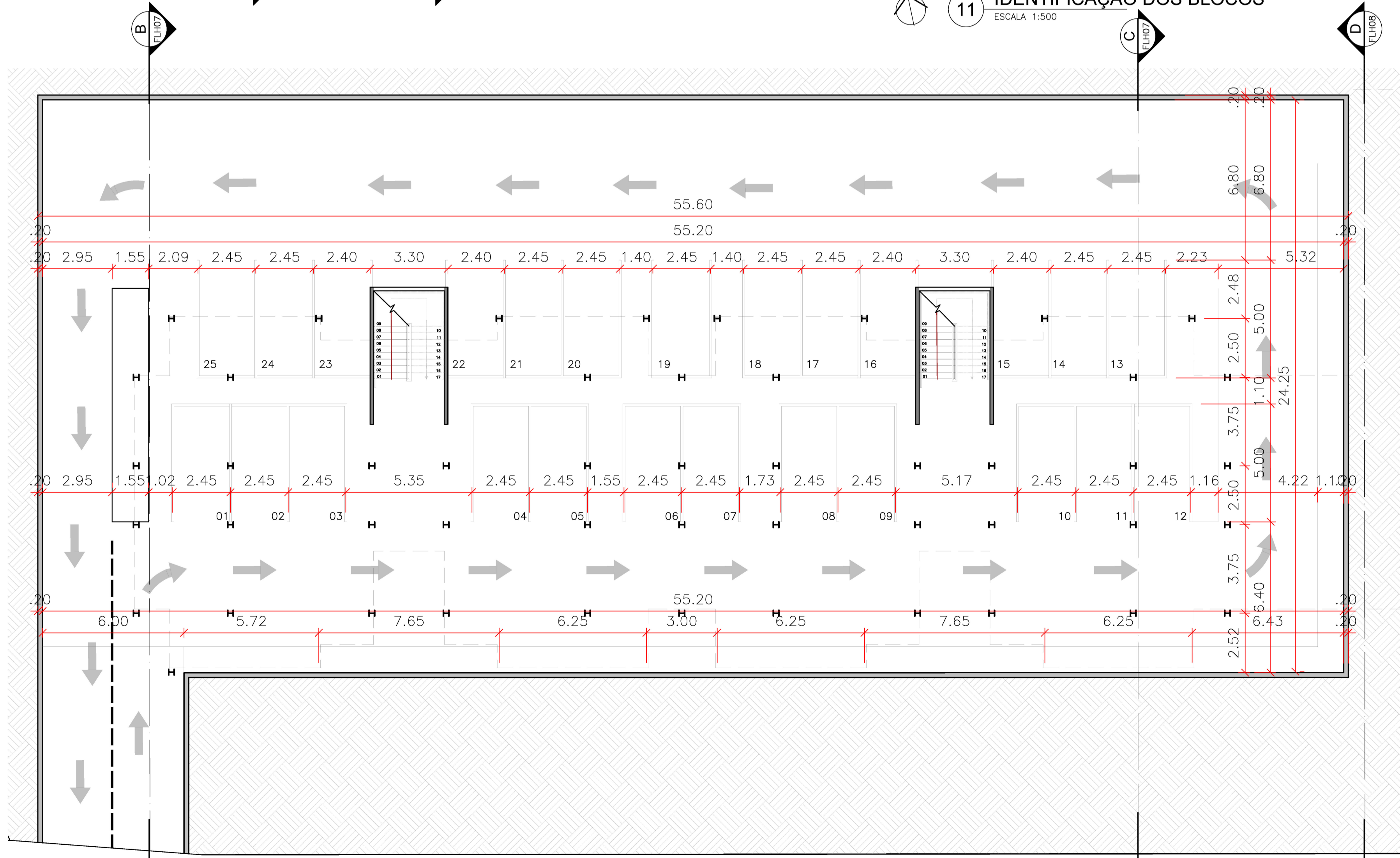
10 ESTACIONAMENTO ESCALA 1:250
