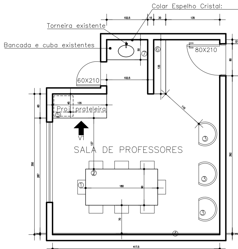
PLANTA BAIXA/ LAYOUT ESC 1: 25
