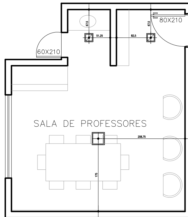
LUMINOTÉCNICO ESC 1: 25
