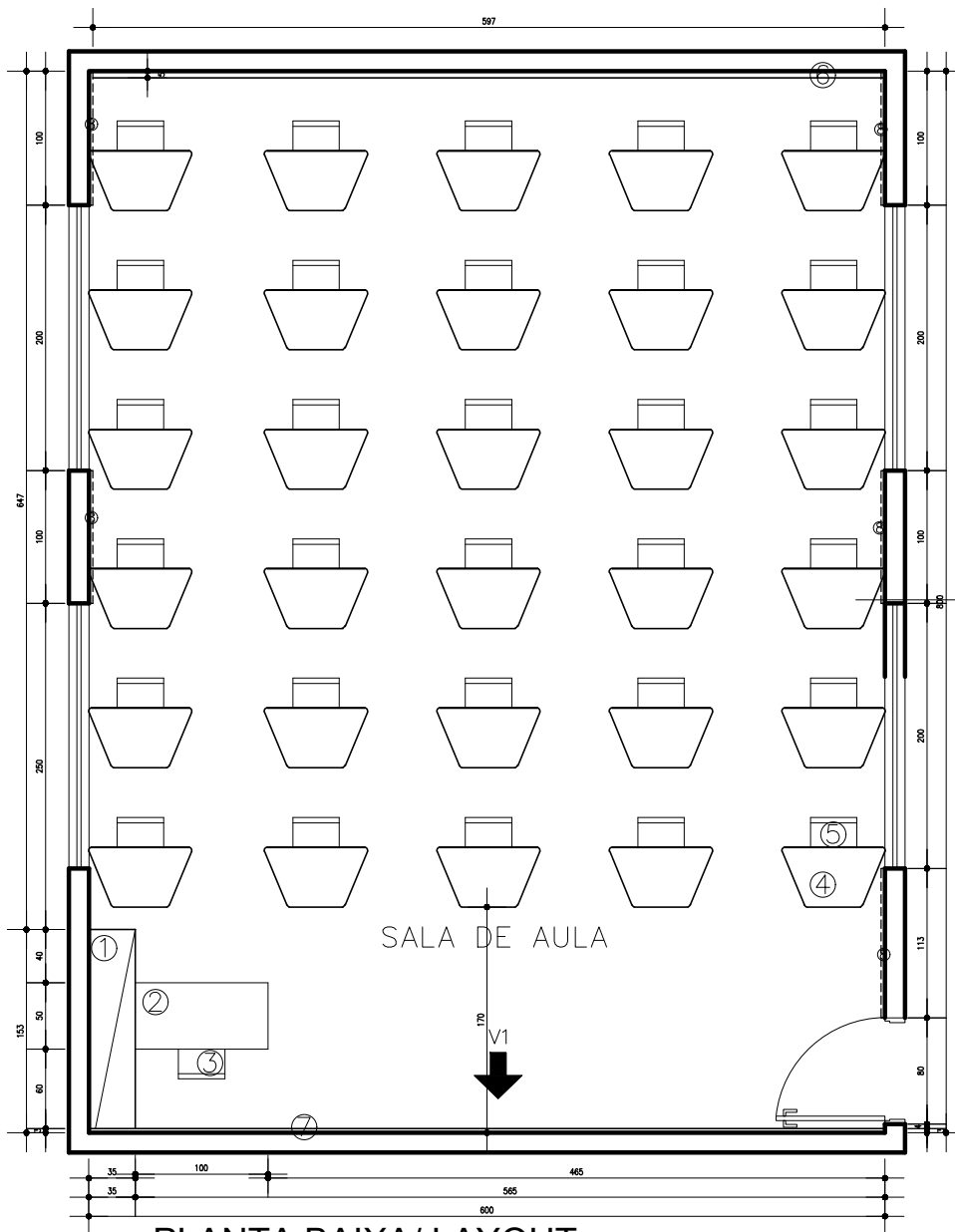
PLANTA BAIXA/ LAYOUT ESC 1: 25
