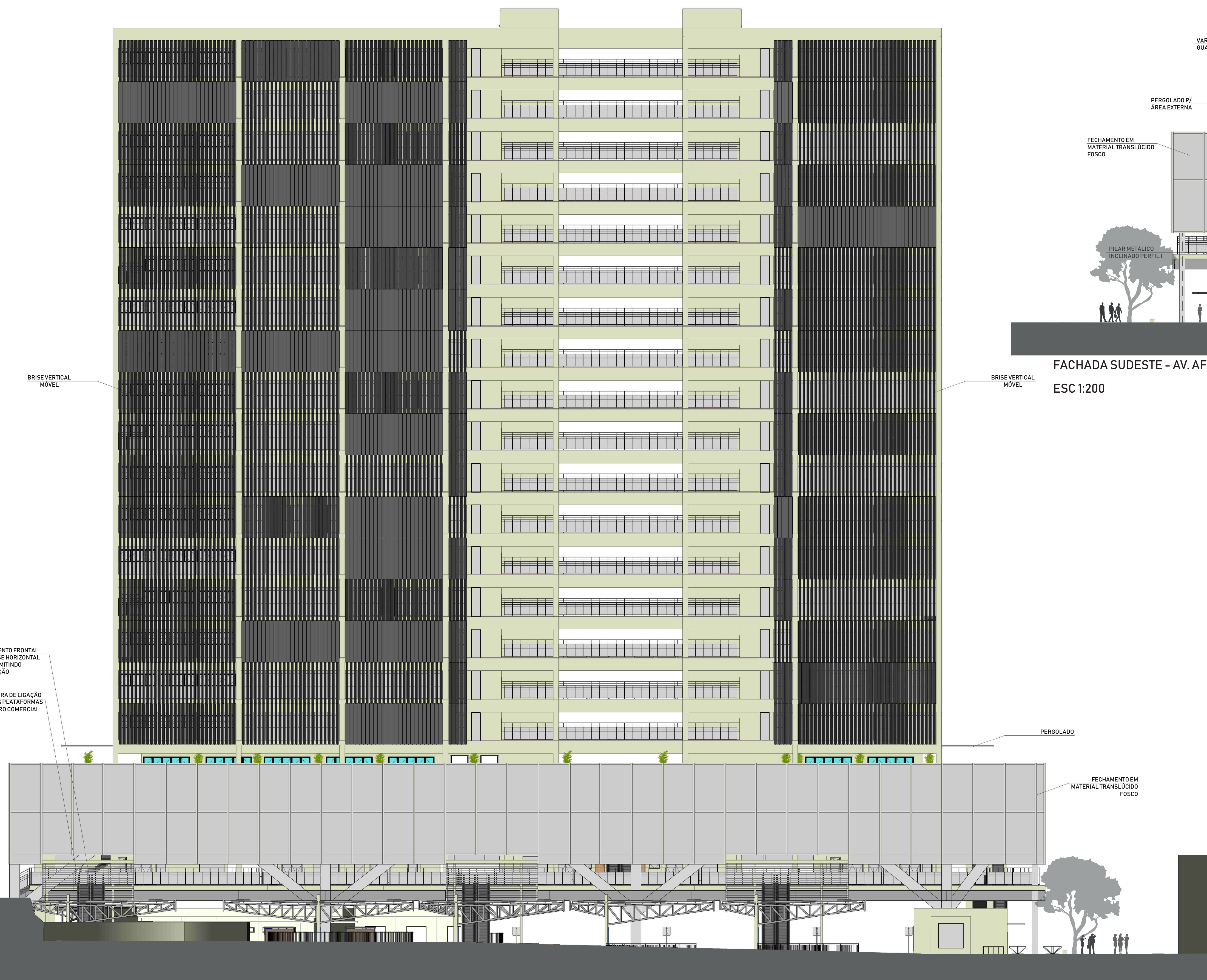
FACHADA NOROESTE - AV. JOÃO PINHEIRO ESC 1:200
