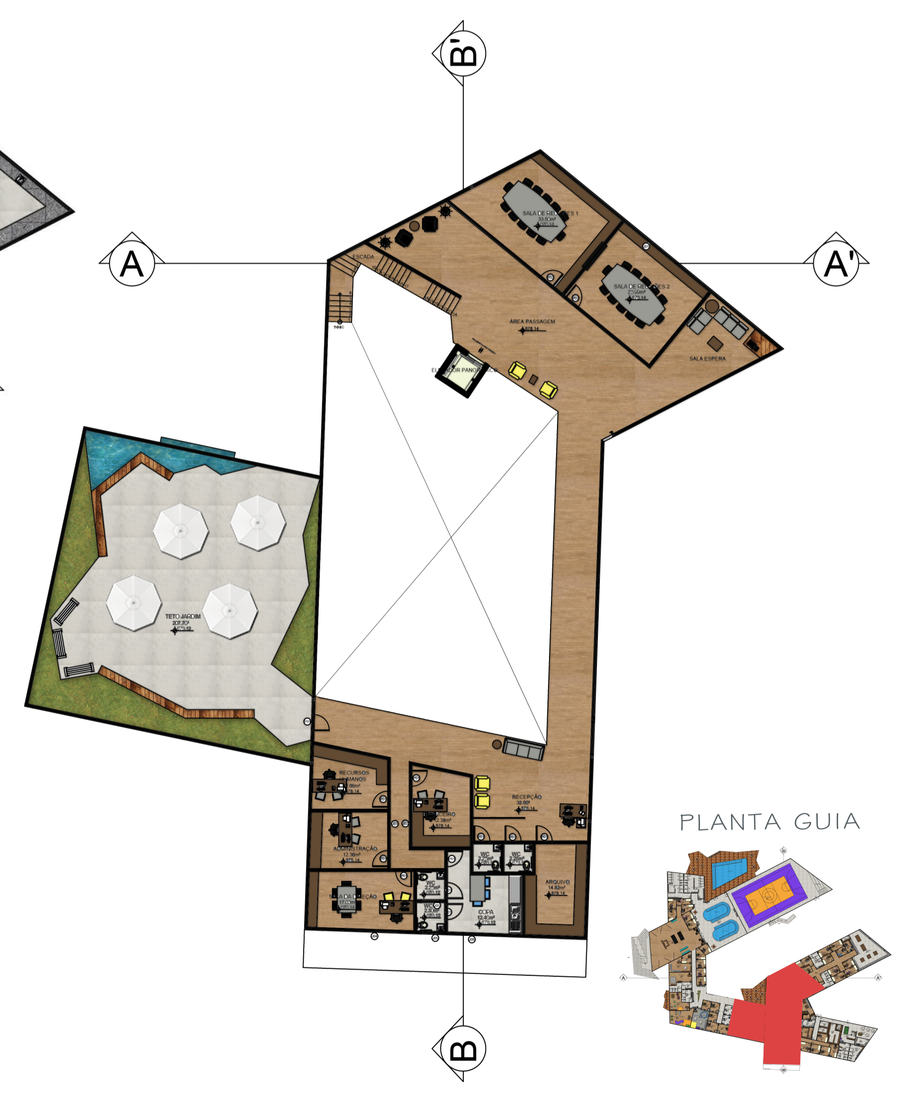
PLANTA PAVIMENTO SUPERIOR
