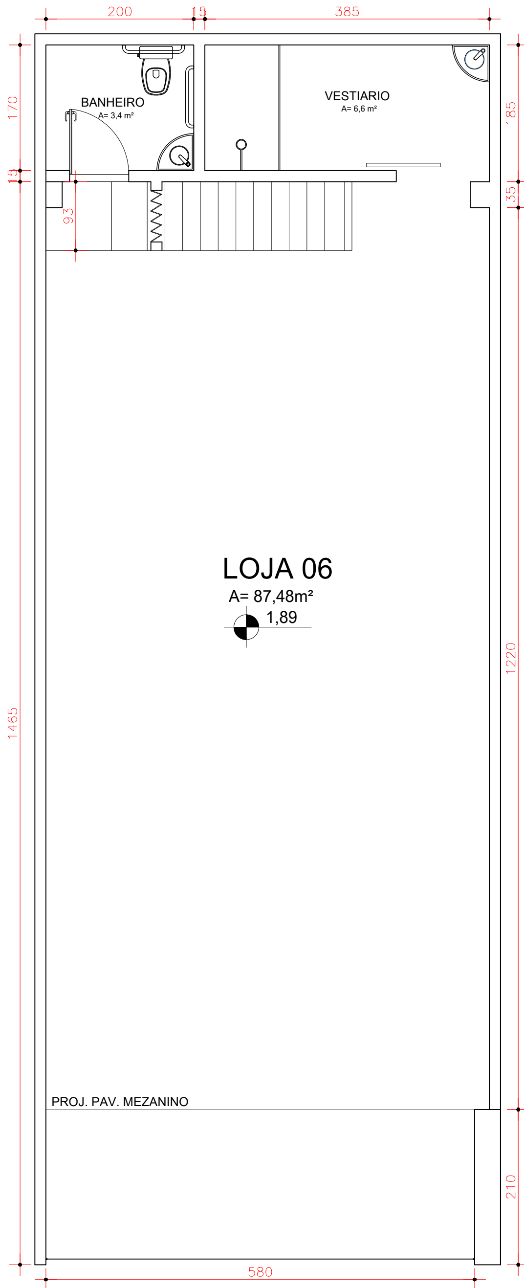
LOJA 06 - PAVIMENTO TÉRREO PLANTA ORIGINAL ESC. 1:50
