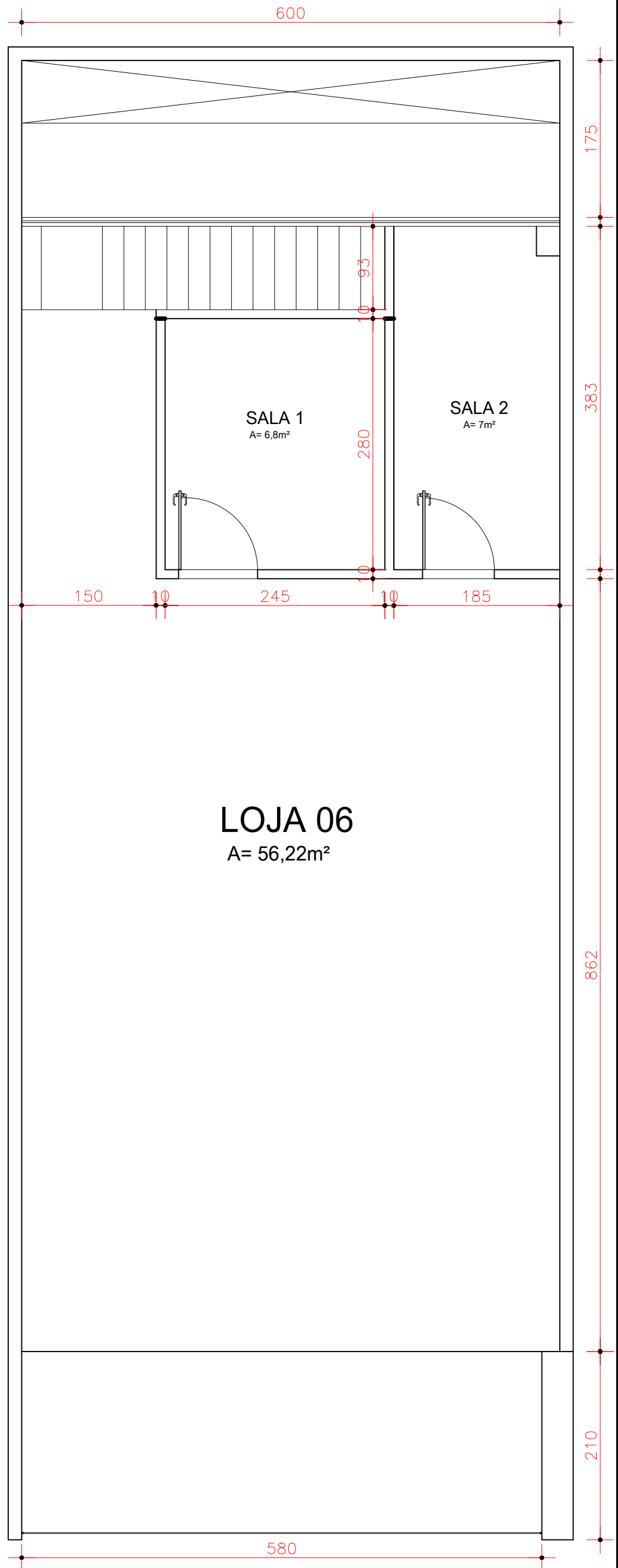
LOJA 06 - PAVIMENTO SUPERIOR PLANTA ORIGINAL ESC. 1:50
