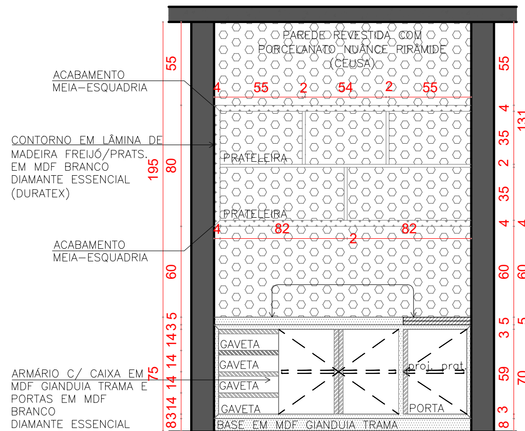
ESCRITÓRIO CORTE BB ESC. 1:25
