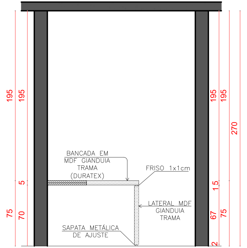
ESCRITÓRIO CORTE CC ESC. 1:25
