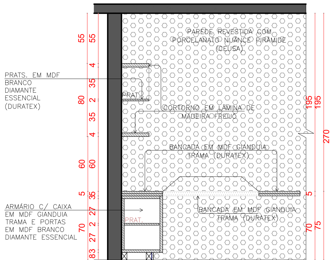
ESCRITÓRIO CORTE AA ESC. 1:25
