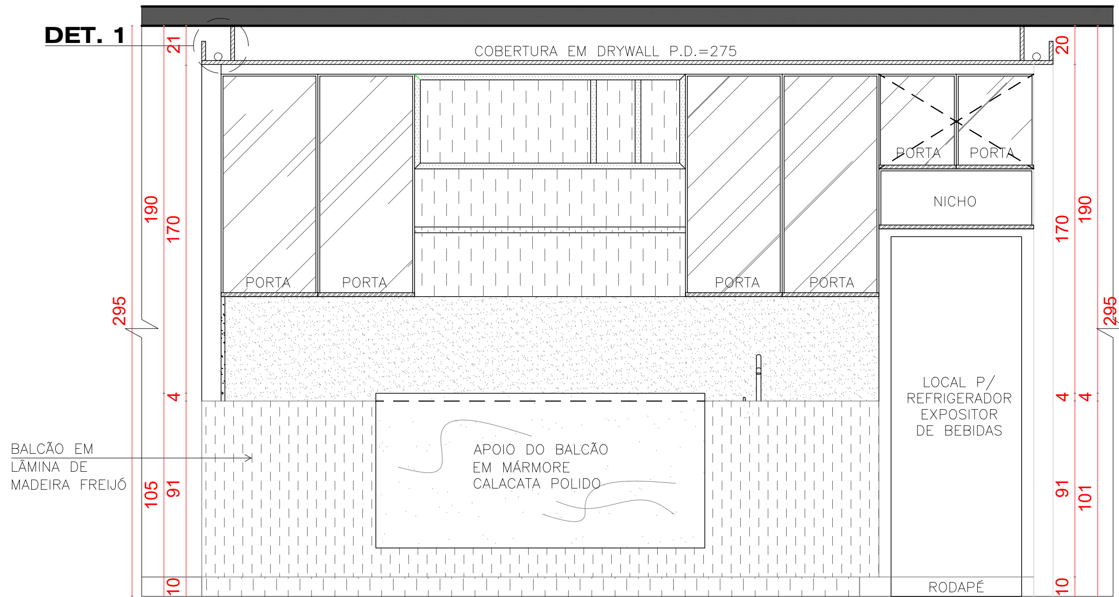
BANCADA CAFÉ VISTA 1 ESC. 1:20
