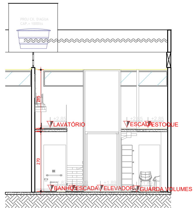
LOJA ESSÊNCIA: MESA POSTA E ETIQUETA CORTE CC ESC. 1:50
